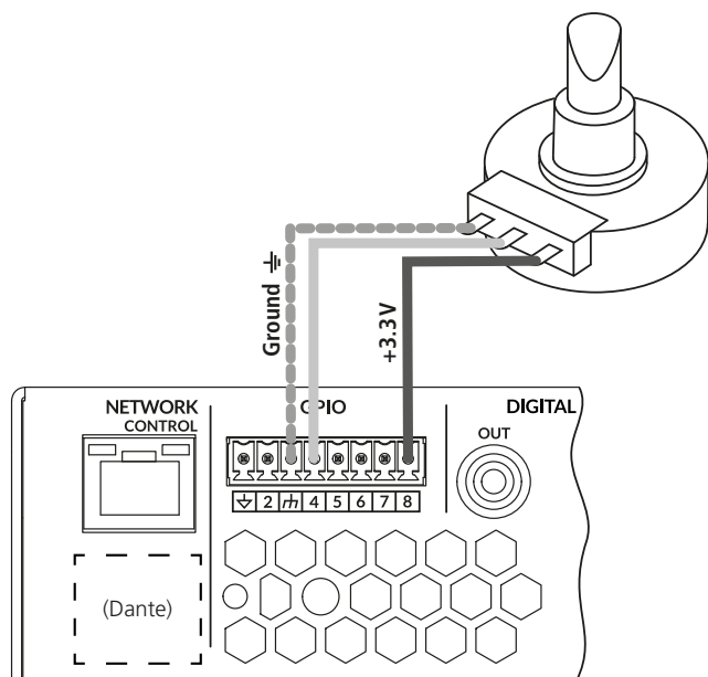
Abb. 5 externer Lautstärkereglер
