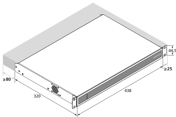
Abb. 4 Belüftungsabstände
