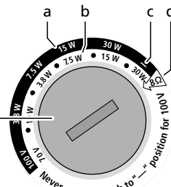
100-V-Betrieb → äußere Skala 70-V-Betrieb → innere Skala dargestellte Schalterposition: 8-Ω-Betrieb
